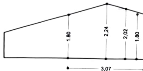
SEZIONE A - A
